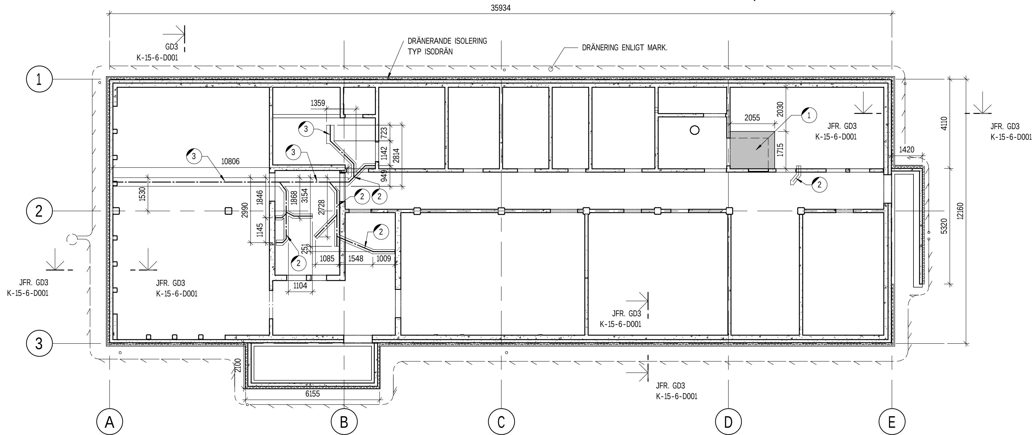
D090 GRUNDPLAN 1 : 100
