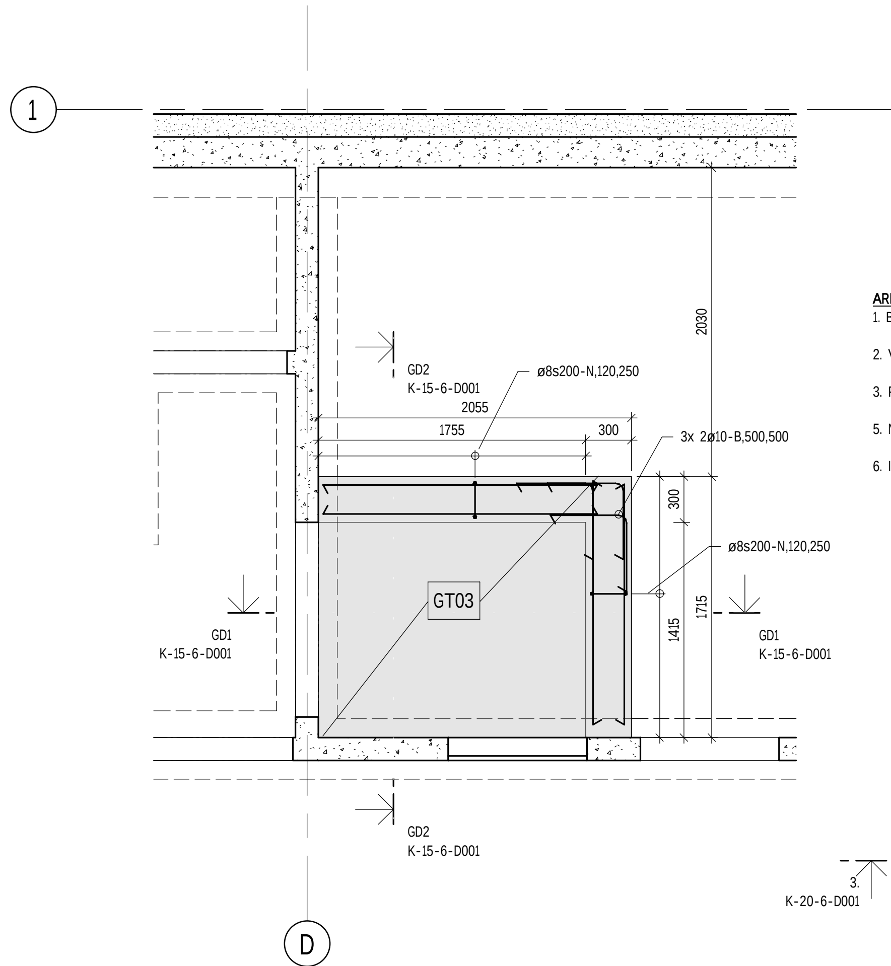
GRUNDPLAN HISSGROP 1 : 25
